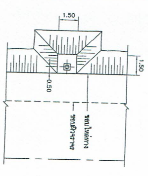
แปลนเสาไฟถนน ติดตั้งบนพื้นดิน
