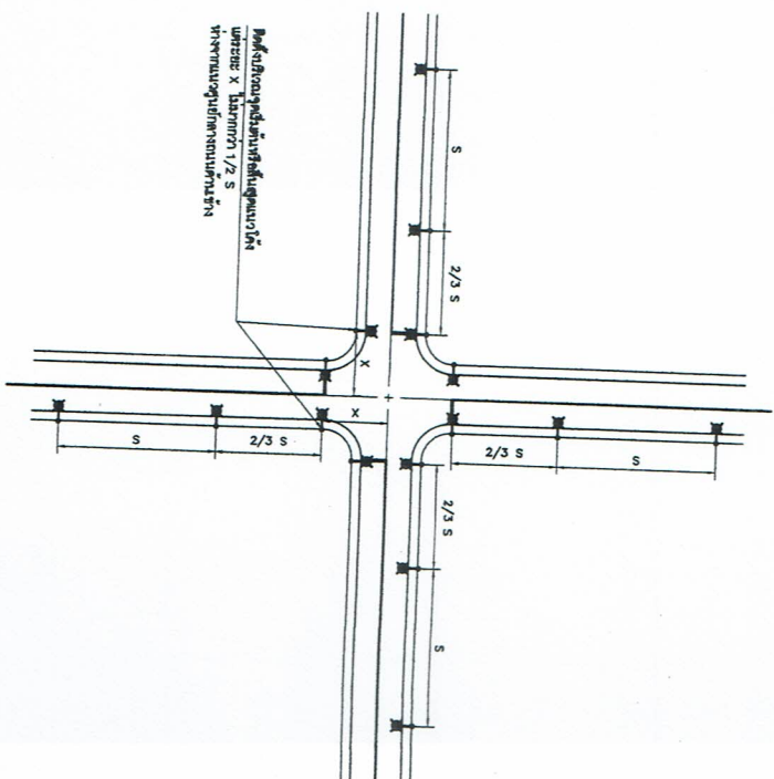
รูปแบบการติดตั้งเสาไฟฟ้าแสงสว่างถนนบริเวณแยก
