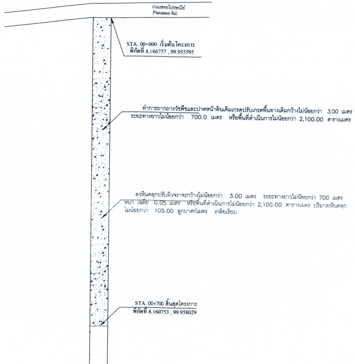
แปลน โครงการปรับปรุงถนนสายสีทอง-สีพริก หมู่ที่ 2 construction plan no scale
