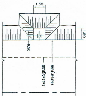
แปลนเสาไฟถนน ติดตั้งบนพื้นดิน ไม่ตั้งงอตามตัว
