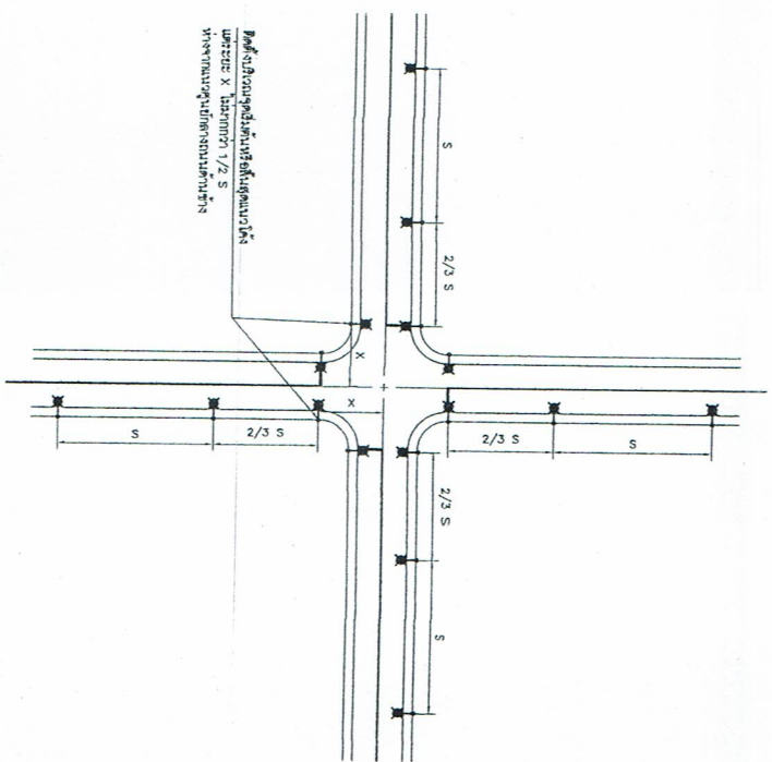
รูปแบบการติดตั้งเสาไฟฟ้าแรงส่งช่วงถนนบริเวณสี่แยก ในเขตเทศบาล
