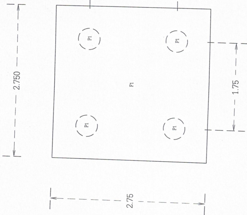
แบบแปลนฐานราก F1 1:25
